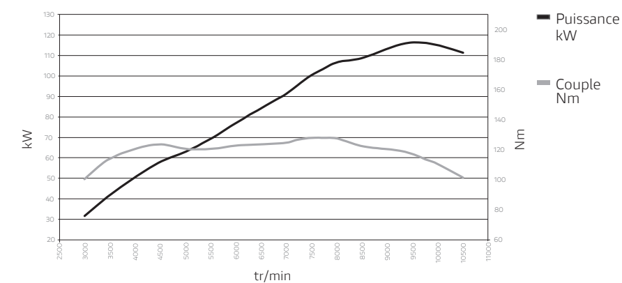
Courbes de puissance / couple
