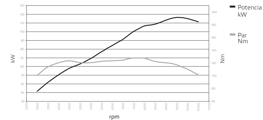
Curvas de potencia / par
